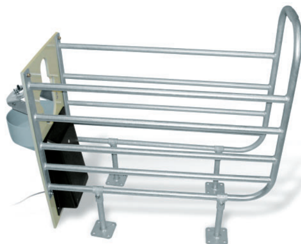
Het drinkstation (B10) met herkenningssysteem CalfScan .
